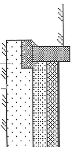
Уплотненный грунт
